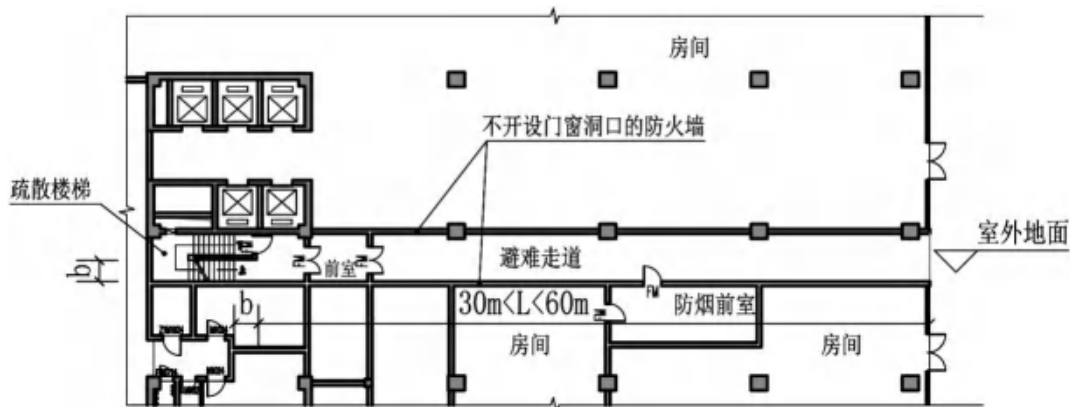
附图 4.2.2 设置避难走道通至室外
