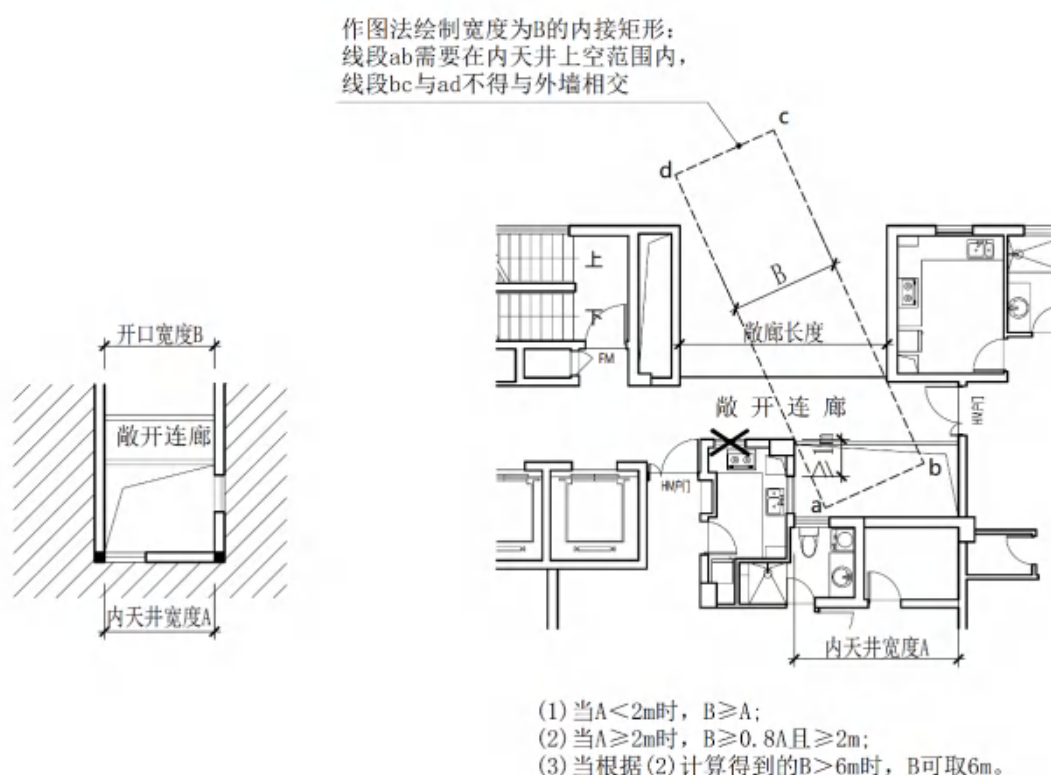
附图 2.3.17 住宅建筑 U 型天井
