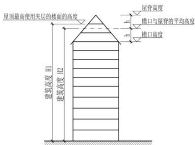
附图 1.1.3 坡屋顶建筑高度计算
