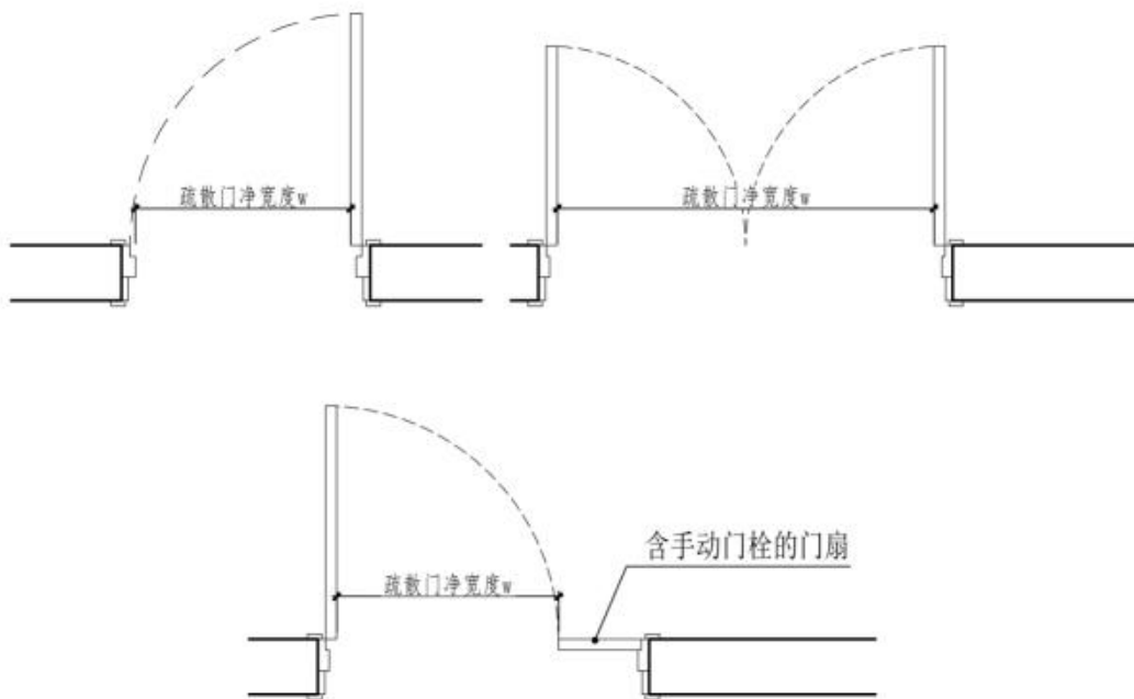
附图 4.1.35 疏散门的净宽计算
