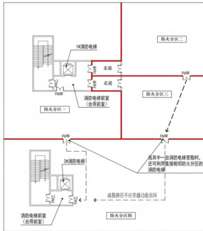
附图 4.3.5 消防电梯的合用
