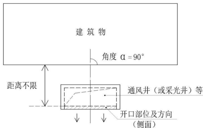
附图 2.3.3 开口背向建筑物
