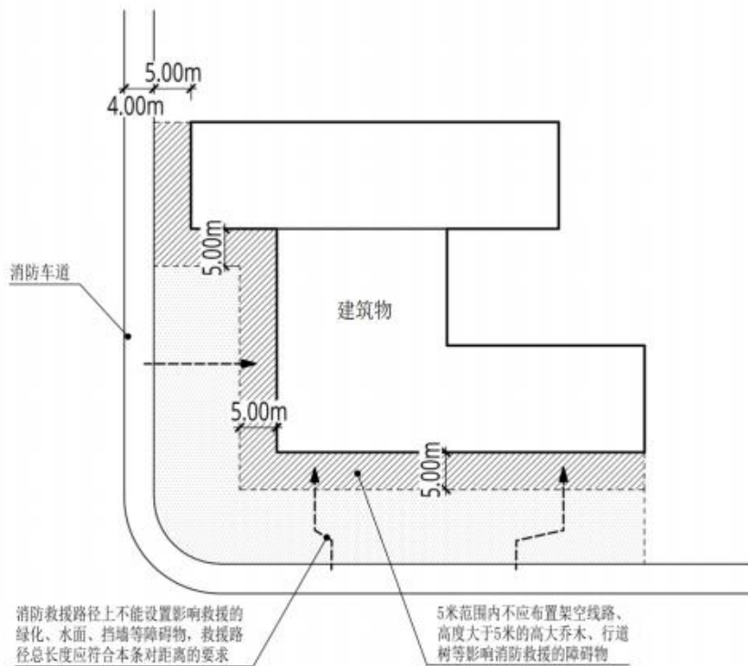
附图 2.1.1 消防车道与建筑之间的障碍物
