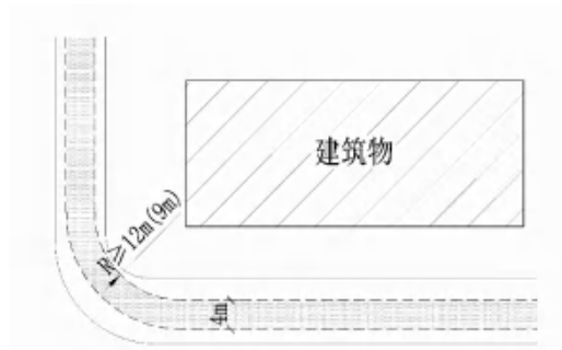
附图 2.1.2 消防车道转弯半径
