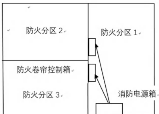
图 6.1.4 多个防火分区多个防火卷帘供电示意图
