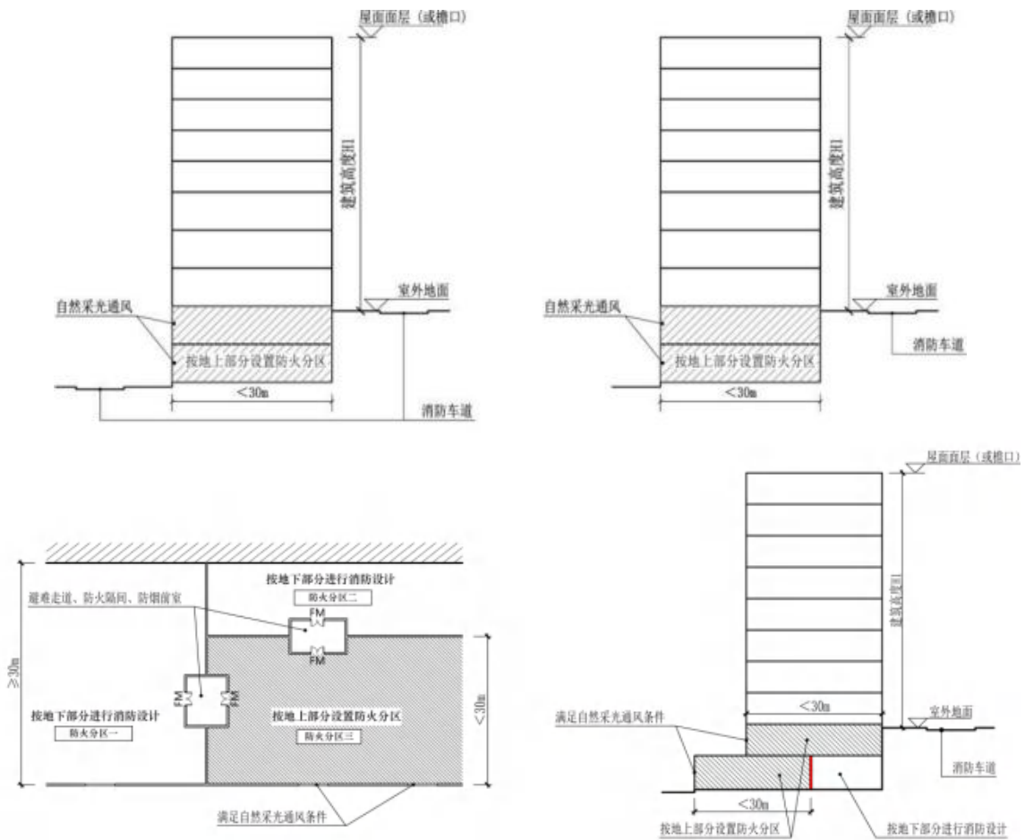
附图 1.2.2-1 按较高的室外地坪起算建筑高度
