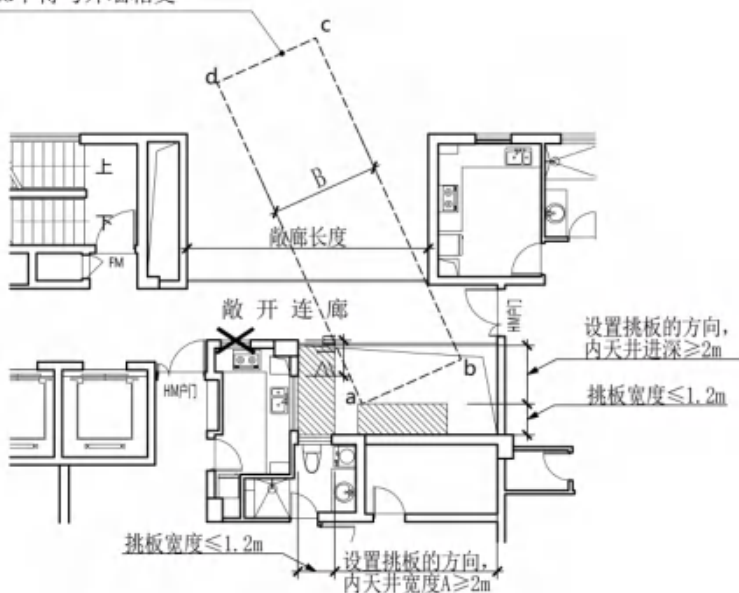
附图 2.3.18 住宅建筑 U 型天井挑板
