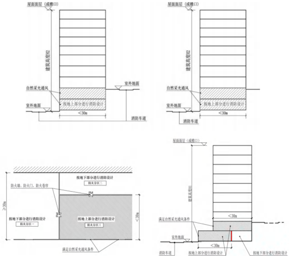
附图 1.2.2-3 按较低的室外地坪起算建筑高度
