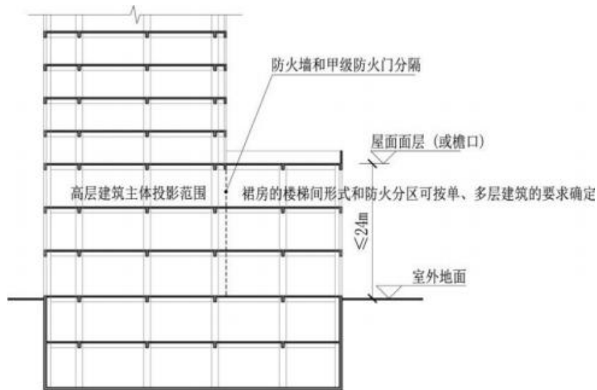
附图 1.5.2 裙房的疏散楼梯形式和防火分区
