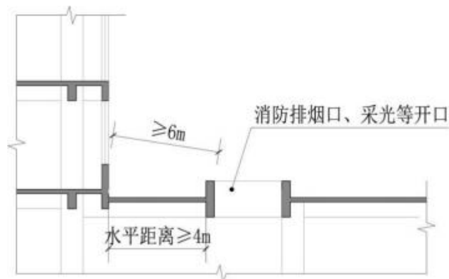
附图 2.3.2 建筑屋顶和地下室顶板开口设置
