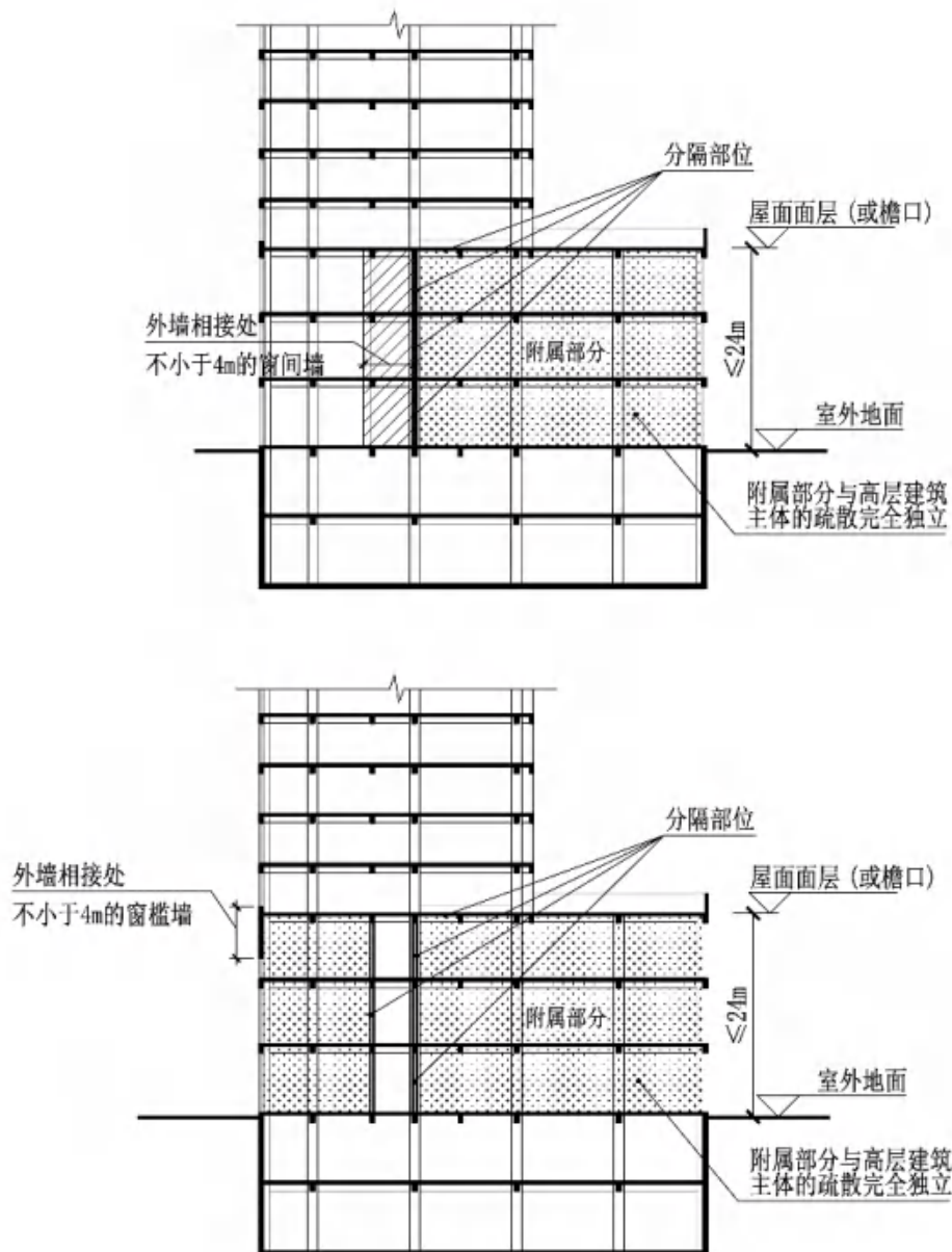
附图 1.5.3 多种功能组合的高层建筑下部的附属部分
